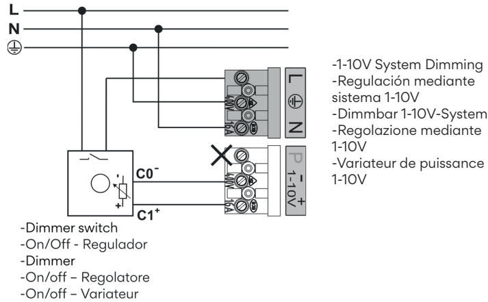
Diagram / Diagrama / Anschlussschema / Diagramma / Diagramme Y
