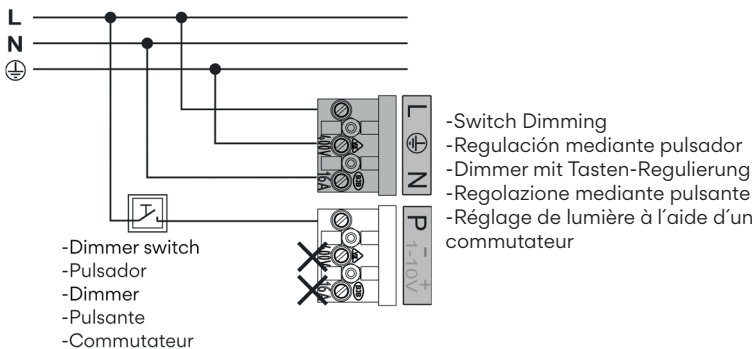
Diagram / Diagrama / Anschlussschema / Diagramma / Diagramme Y
