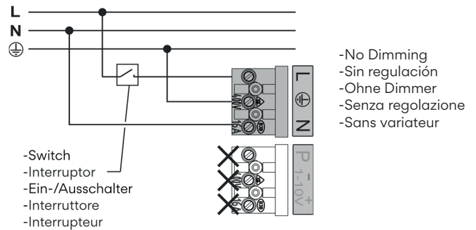
Diagram / Diagrama / Anschlussschema / Diagramma / Diagramme Z
