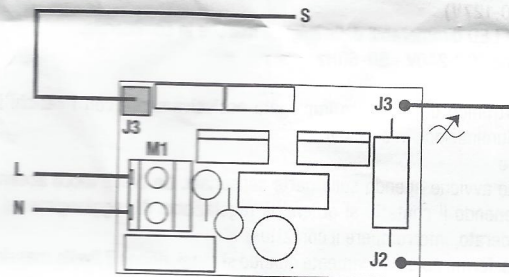
Fig. 2 - Schema di collegamento - Wiring diagram
