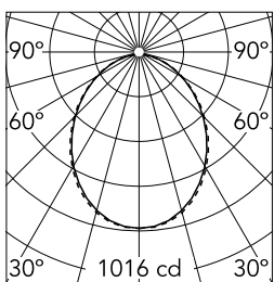
Luminous flux luminaire 2364 lm
