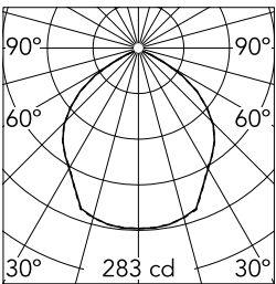
Luminous flux luminaire 631 lm
