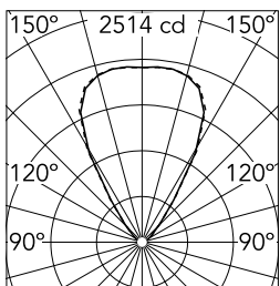
Luminous flux luminaire 2574 lm
