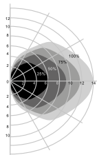
Ansbereich Wandmontage (Einheit: m) Empfohlene Montagehöhe: 1 - 1.8m
