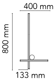
F18110_24W_LED_COORDINATES_W2
