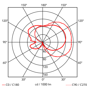
F18110_24W_LED_COORDINATES_W2
