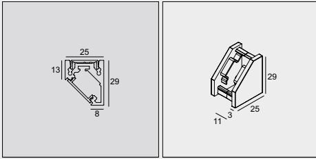
FTL25 T - PROFILE
