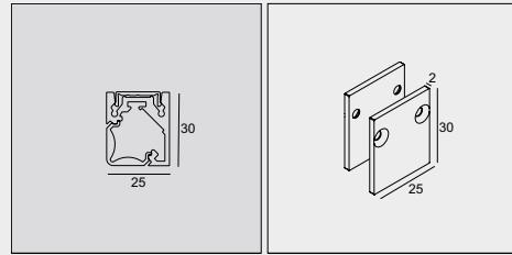
FTL25 TP - PROFILE
